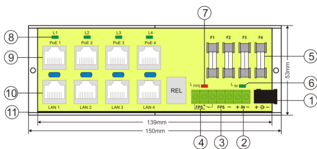
Rys. 1. Rysunek modułu.
